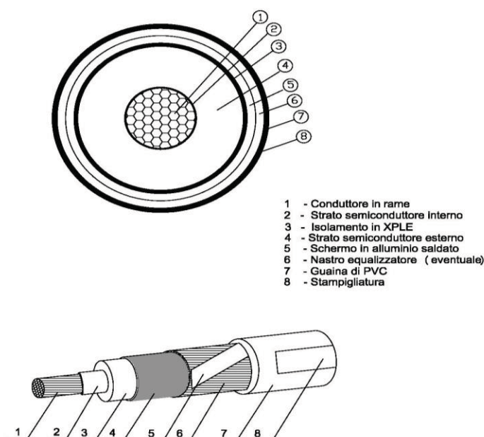
Figura 1: Schema tipo del cavo 150 kV
