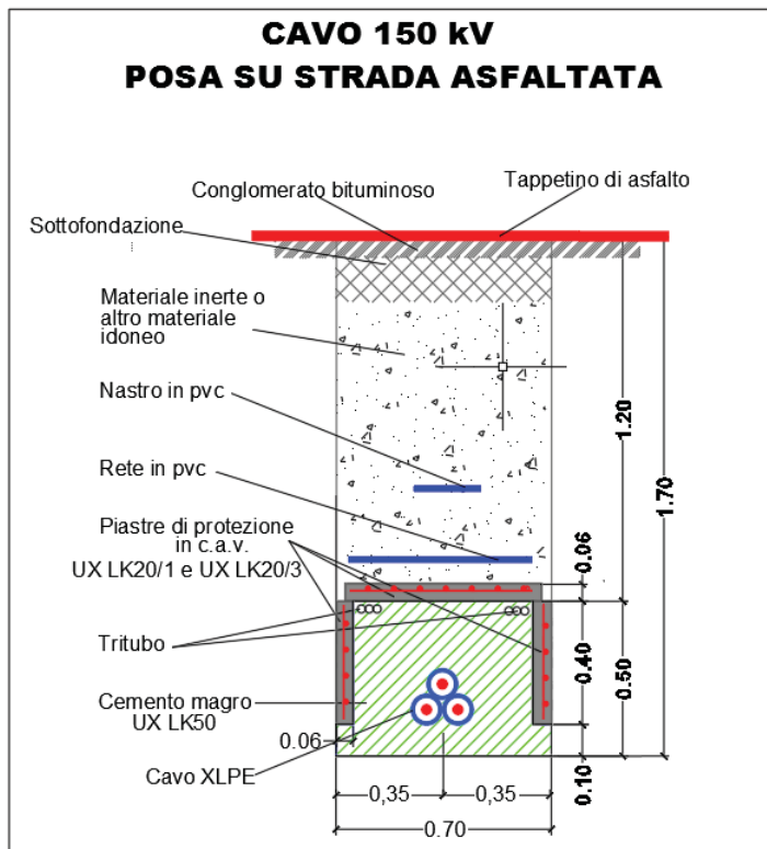
Fig 2 Posa cavo 150 kV "SE 30/150 kV – C.P. Balabritto"
