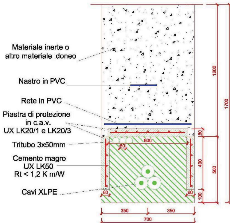
Fig 2 Posa cavo 150 kV "SE 30/150 kV – C.P. Balabritto"
