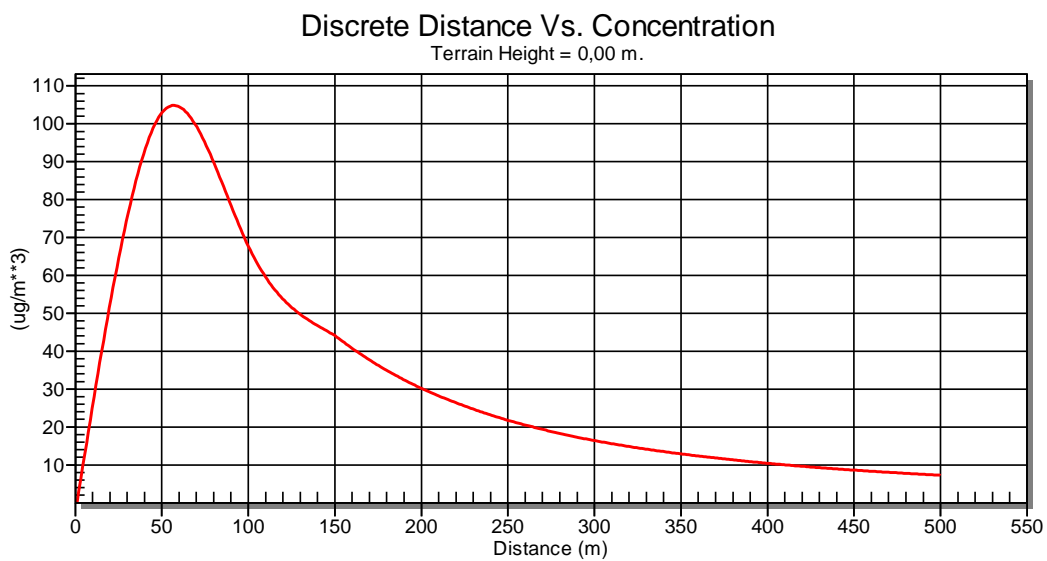
Figura 7-B: Concentrazione NO2 vs Distanza Sorgente
