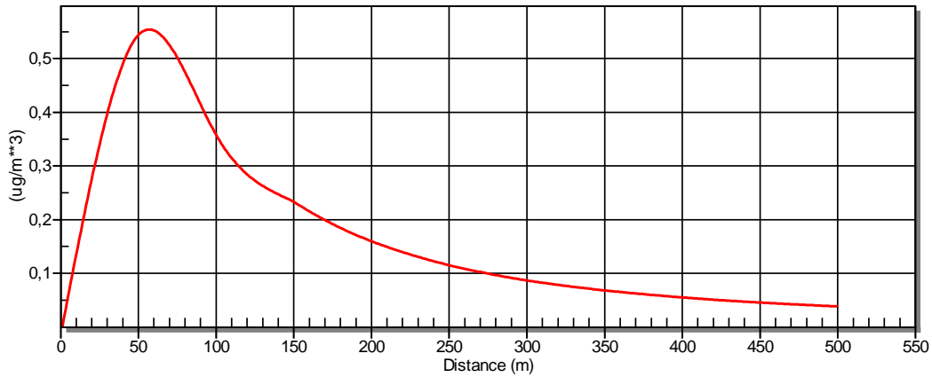
Figura 7-C: Concentrazione SO2 vs Distanza Sorgente
