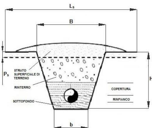
Figura 4-A: Sezione tipo dello scavo per l'alloggiamento delle condotte
