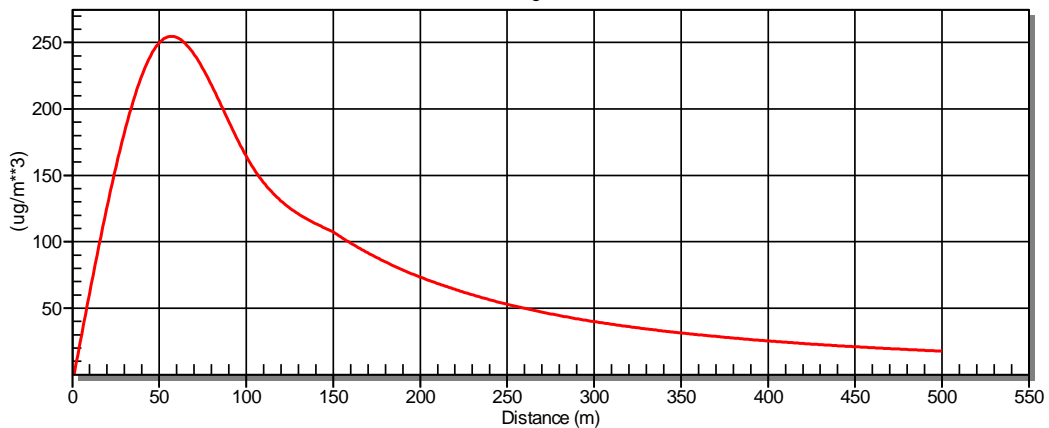
Figura 7-D: Concentrazione CO vs Distanza Sorgente
