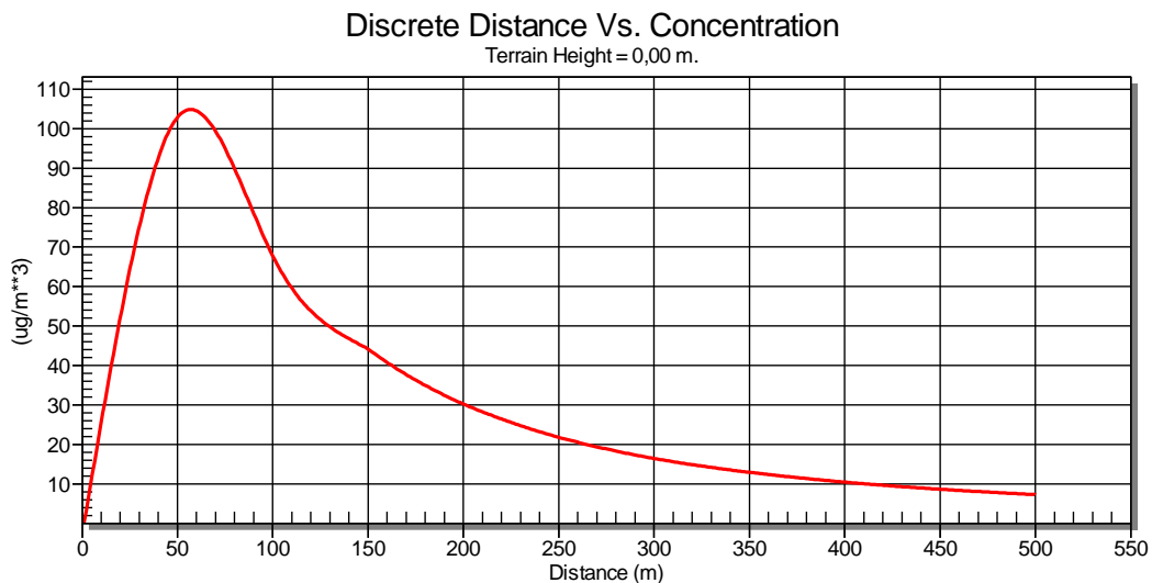
Figura 7-A: Concentrazione PM10 vs Distanza Sorgente
