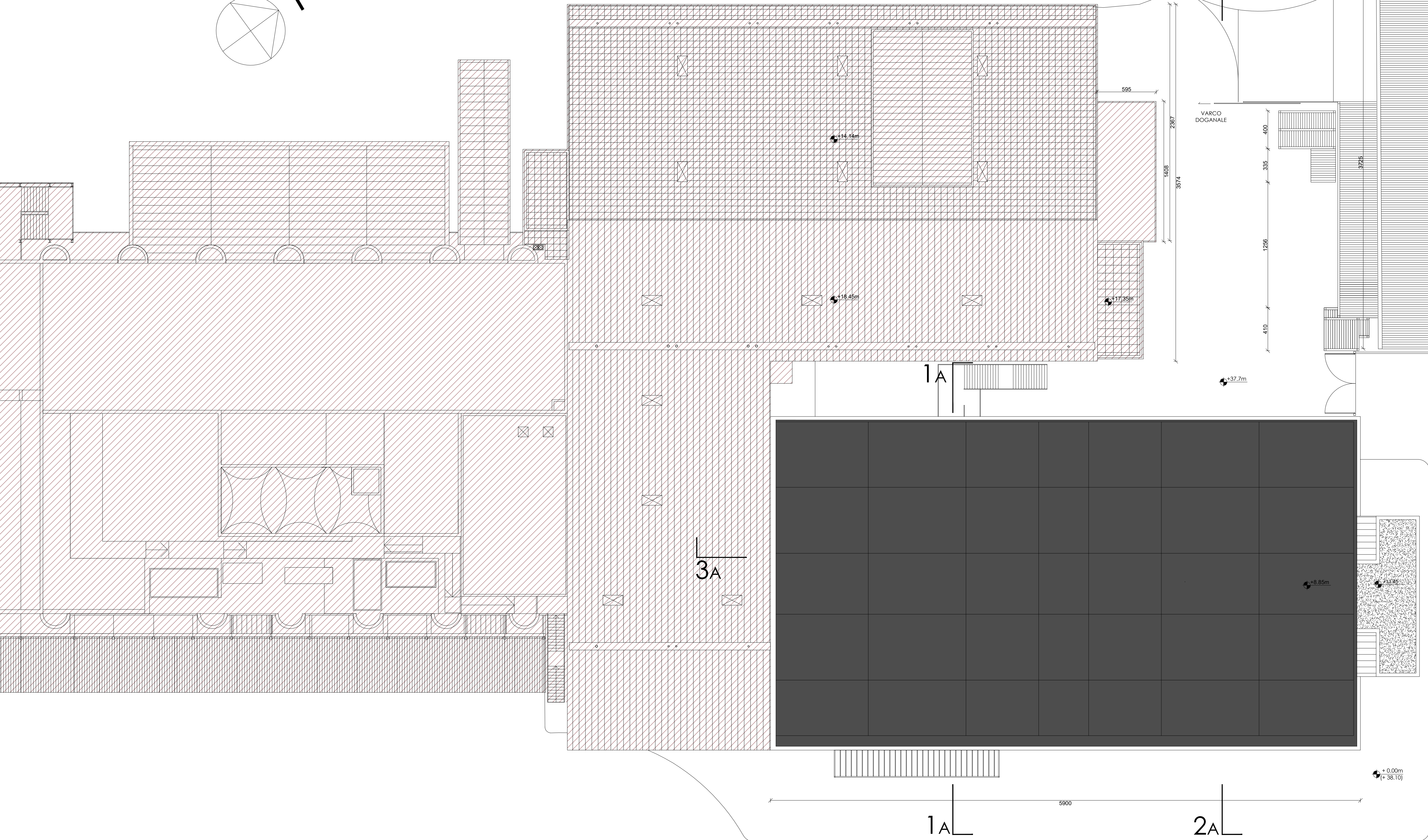
PIANTA DELLE COPERTURE 1:200
