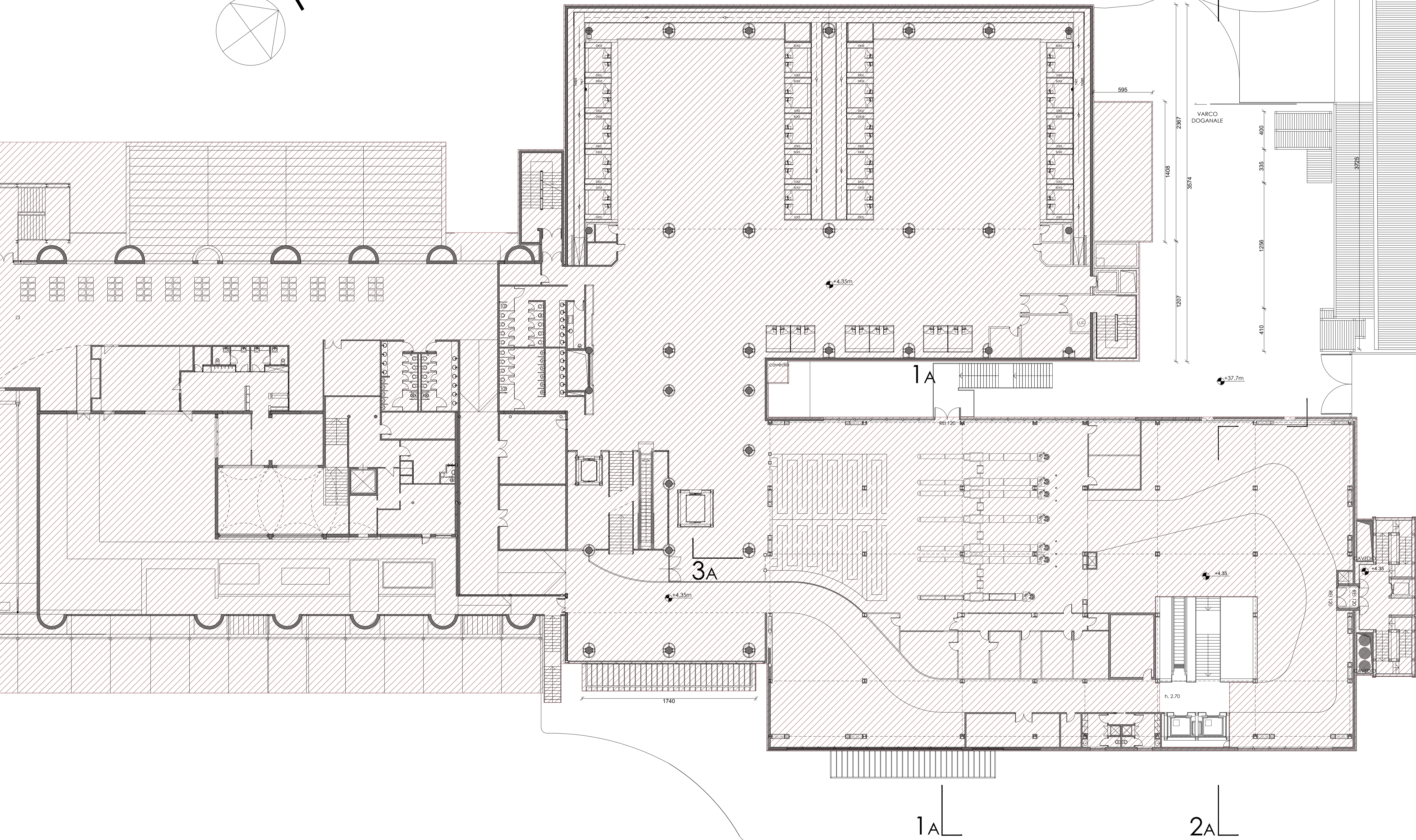
PIANTA PIANO PRIMO 1:200
