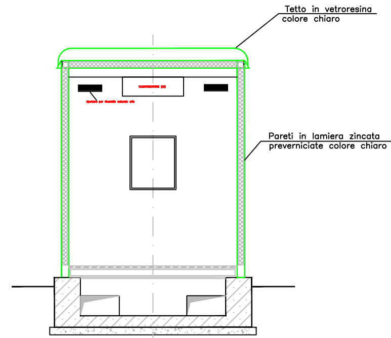
SEZIONE "W-W"
