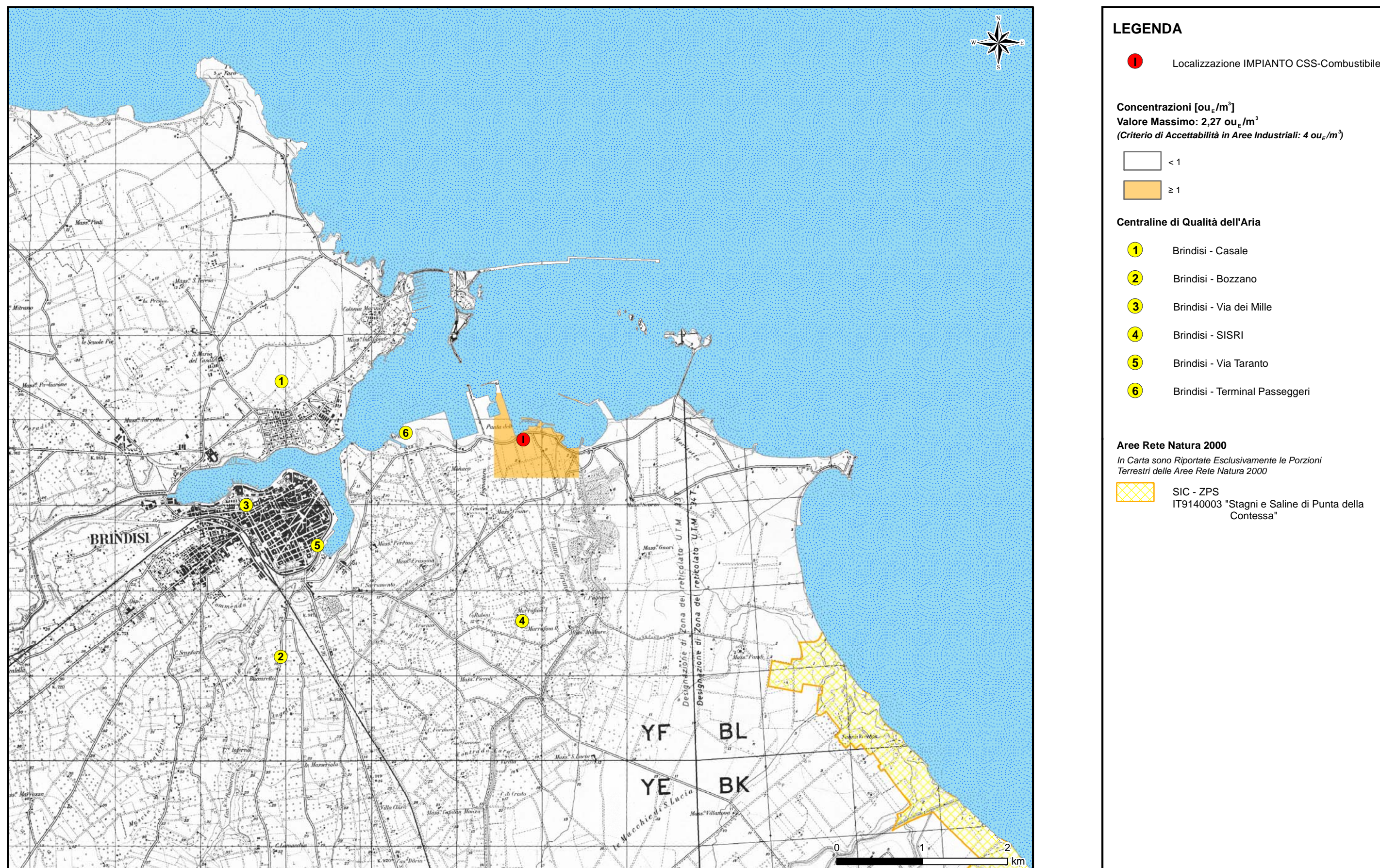
Figura A4.5.1d 98° Percentile delle Concentrazioni di Picco di Odore - Impianto di Produzione CSS Combustibile + CTE Edipower in Assetto co-Combustione Carbone CSS-Combustibile - Scenario Portata Media
