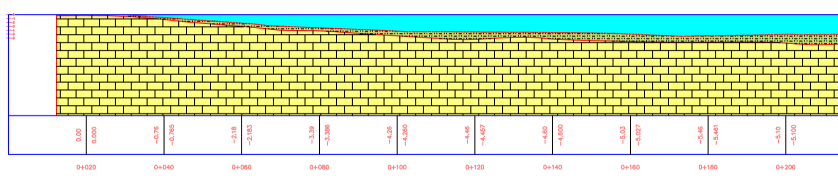
Sezione EE' PROFILE
